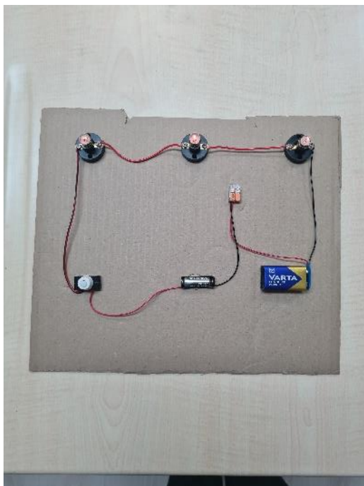
Circuit serie realizat de elevul Olteanu David Alexandru, clasa a VI-a.
