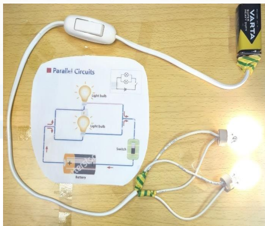
Circuit paralel realizat de elevii Radu Raisa și Stoicescu Eric Mihai, clasa a VI-a.
